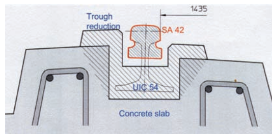
Fig. 6: Low noise SA 42
