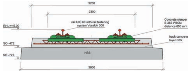
Fig. 2: Rheda 2000
